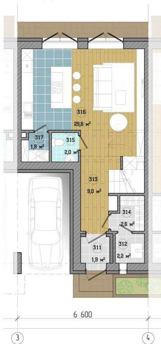
Будинок 5 Планувальні рішення 1-го поверху
