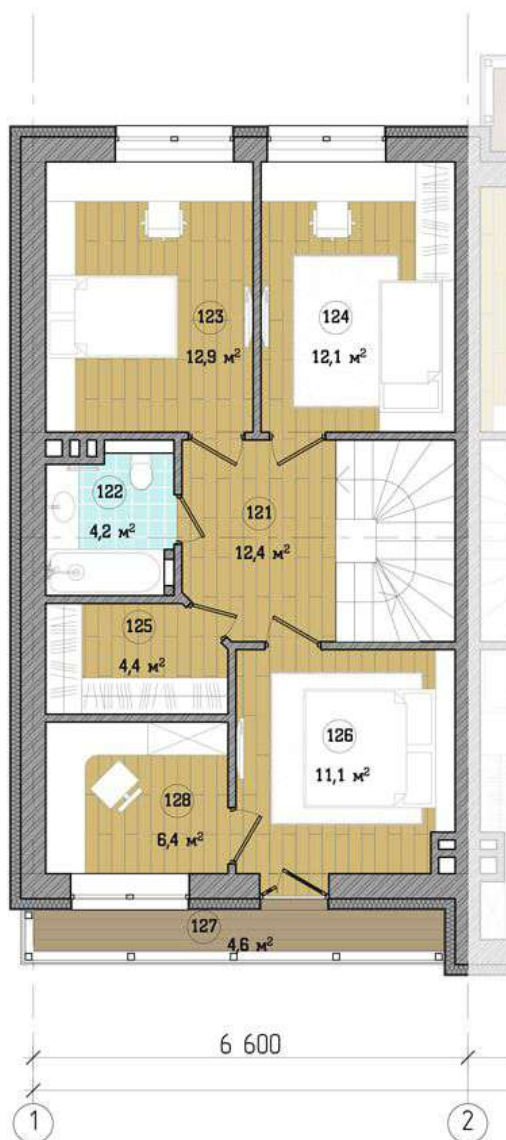
Будинок 7 Планувальні рішення 2-го поверху
