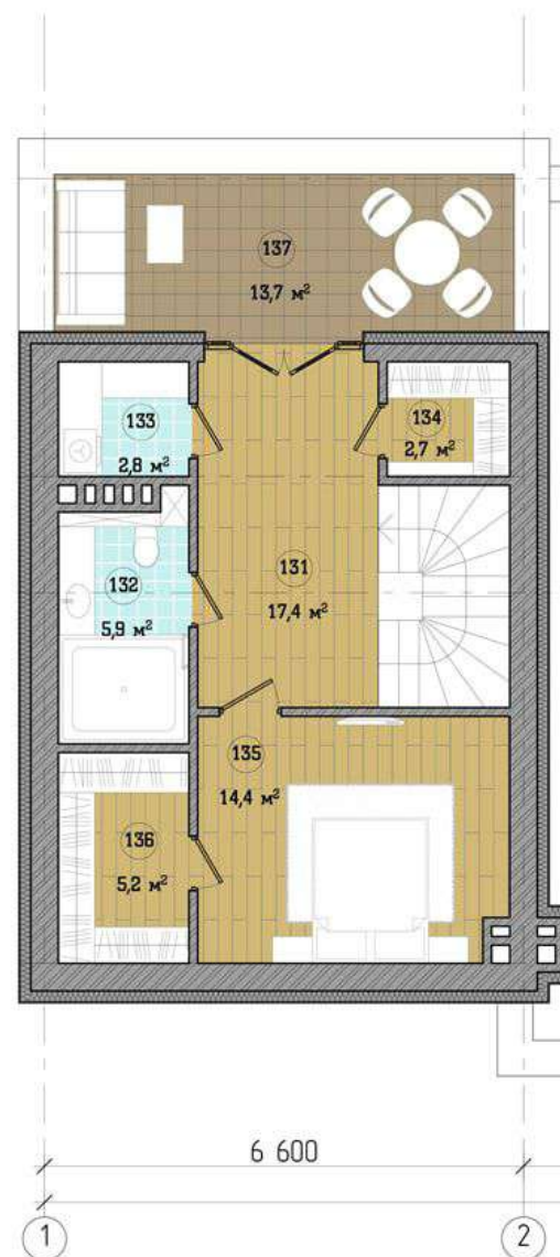
Будинок 7 Планувальні рішення 3-го поверху
