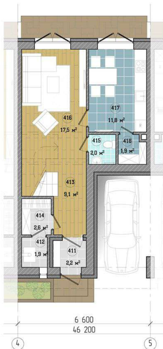
Будинок 4 Планувальні рішення 1-го поверху
