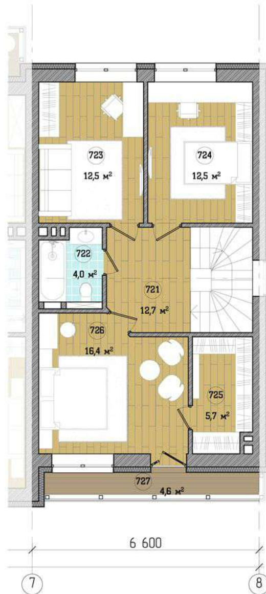
Будинок 1 Планувальні рішення 2-го поверху
