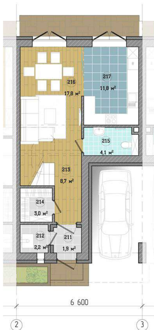
Будинок 6 Планувальні рішення 1-го поверху
