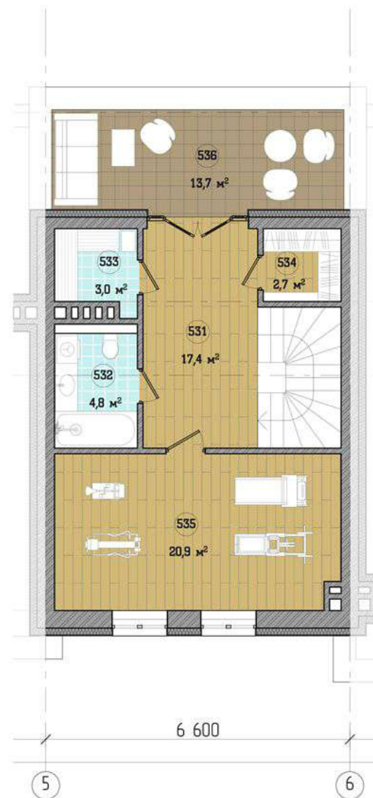
Будинок 3 Планувальні рішення 3-го поверху
