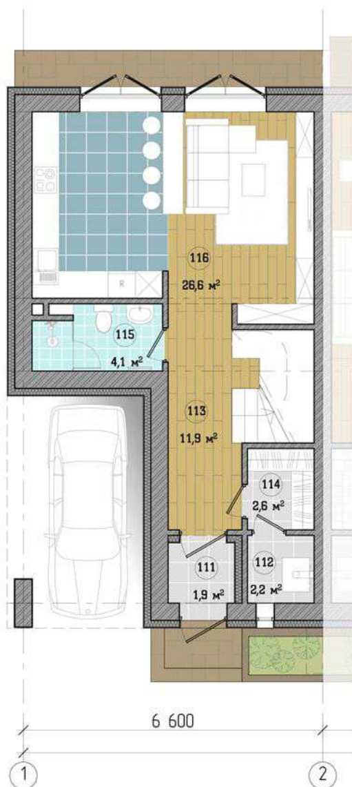
Будинок 7 Планувальні рішення 1-го поверху
