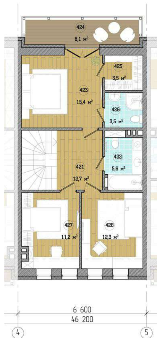
Будинок 4 Планувальні рішення 2-го поверху
