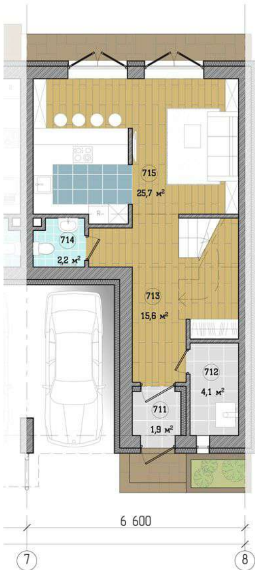
Будинок 1 Планувальні рішення 1-го поверху
