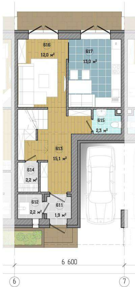
Будинок 2 Планувальні рішення 1-го поверху
