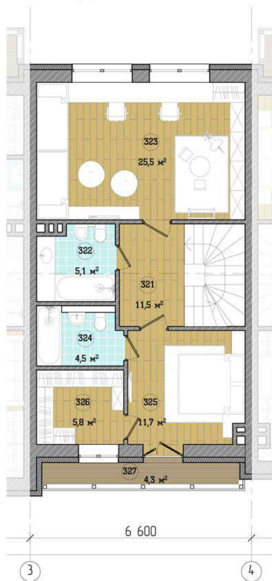
Будинок 5 Планувальні рішення 2-го поверху
