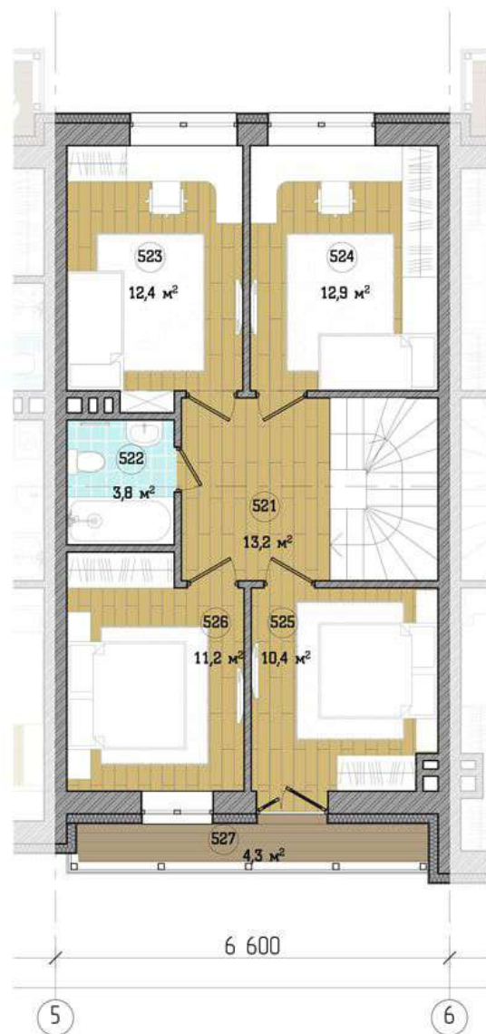
Будинок 3 Планувальні рішення 2-го поверху
